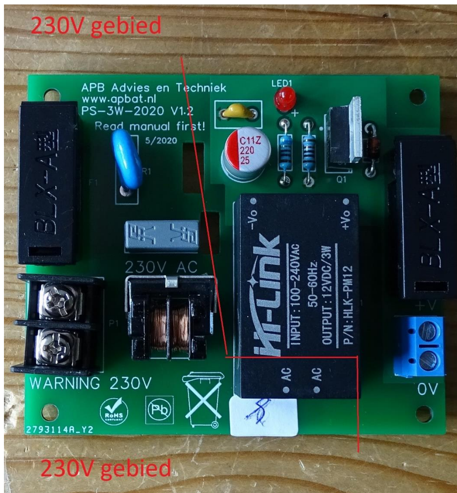
Figuur 1: indicatie 230V gebied gezien vanaf de bovenzijde van de print.
